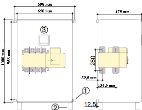
(1) Pattes de fixation murale jusqu'à 400 A. (2) Pieds de réhausse à partir de 630 A (ajouter 200 mm à la cote H, pour les pieds). (3) Interfaces ATyS D10 ou D20 (option)
