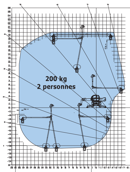
ROTATION SUR STABILISATEURS DEPLOYES AVEC SYSTEME 3 D ZONE DE TRAVAIL EN NEGATIF
