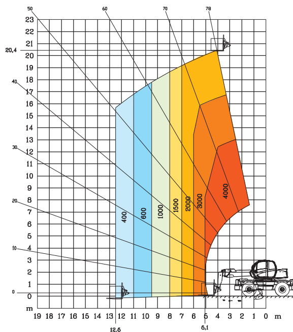
ROTATION SUR STABILISATEURS DEPLOYES AVEC TREUIL 5 T
