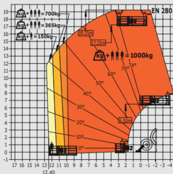
Machine sur stabilisateurs avec nacelle (versions MT 1840 A et MT 1840 HA)
