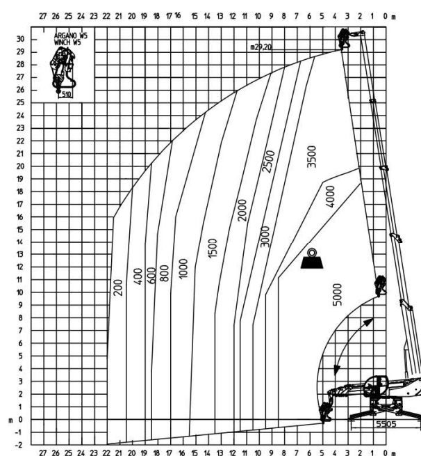
ABAQUE DE CHARGE TREUIL 5t W5 POSITION LATÉRALE AVEC STABILISATEURS
