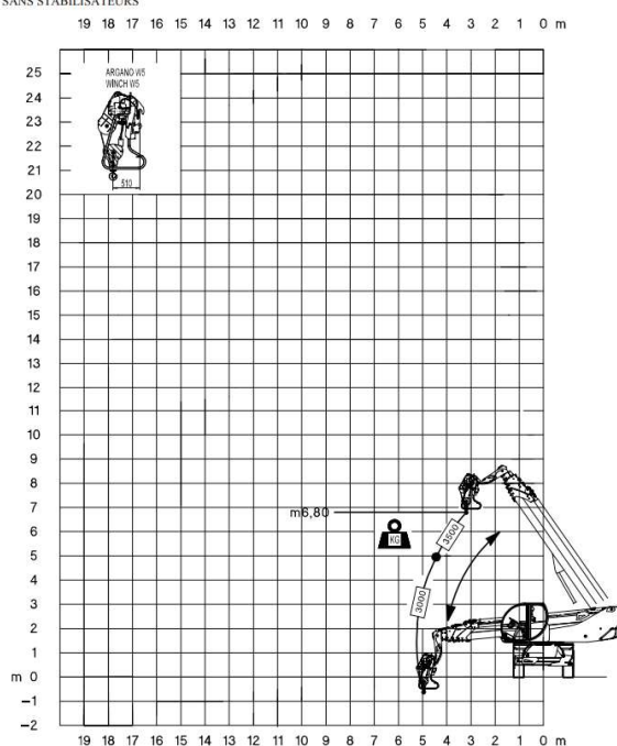
ABAQUE DE CHARGE TREUIL 5t W5 POSITION LATÉRALE SANS STABILISATEURS
