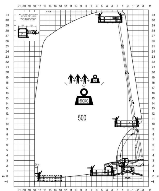
Abaque de charge Panier nacelle 500kg longueur panier 2.35m, 3.54m ou 4.7m
