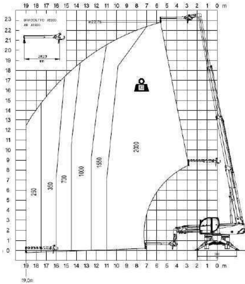
Abaque de charge avec potence courte 5t H5 Position latérale sans stabilisateurs
