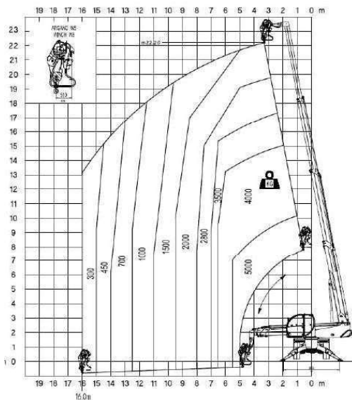
Abaque de charge avec Treuil courte 5t H5 Position latérale avec stabilisateurs
