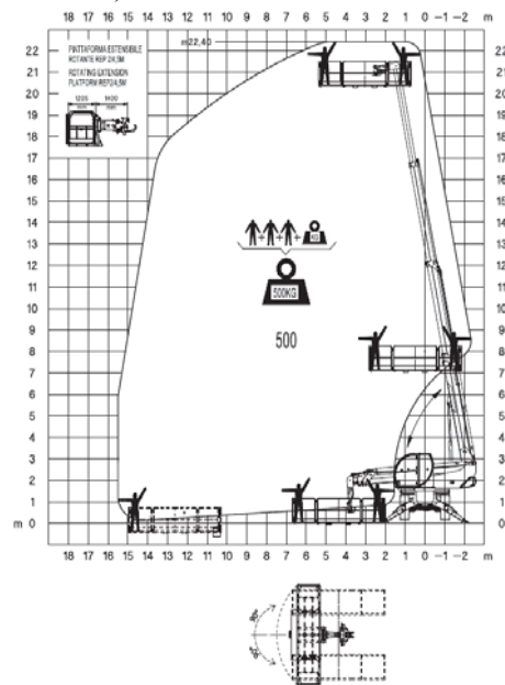
Abaque de charge Panier nacelle 500kg longueur panier 2.35m, 3.54m ou 4.7m
