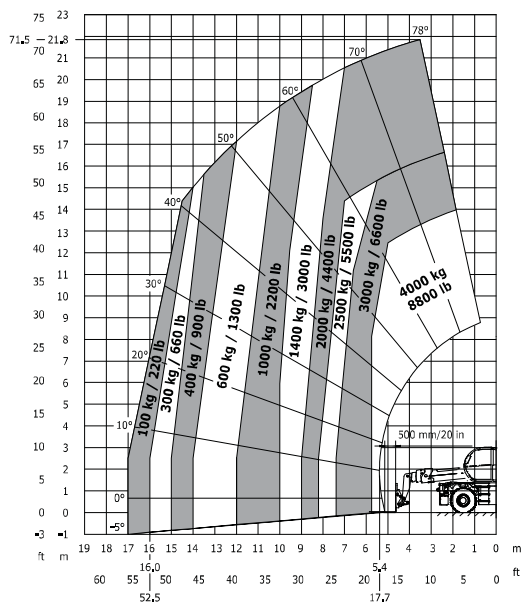
Frontal sur pneus avec fourches
