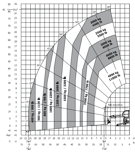
Rotation sur stabilisateurs déployés avec fourches
