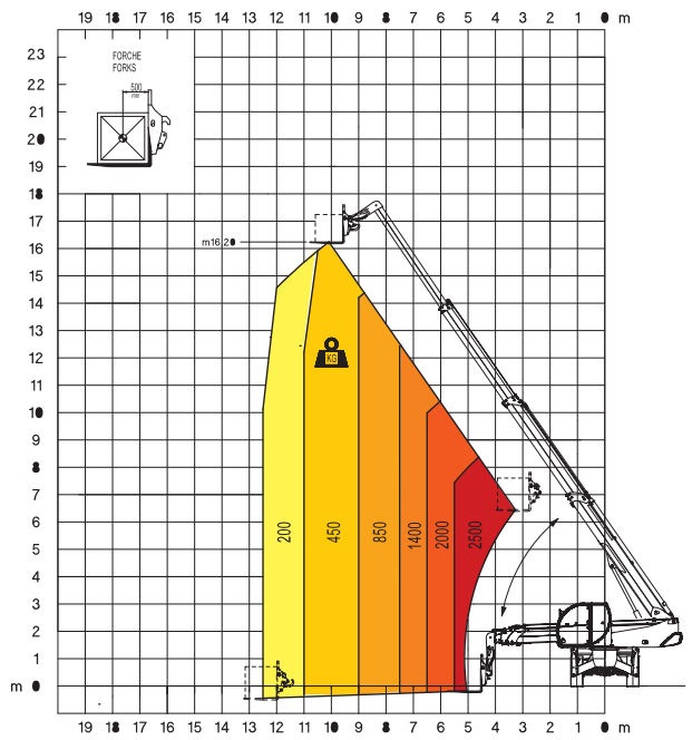
Abaque de charge avec fourches Position frontale sans stabilisateurs
